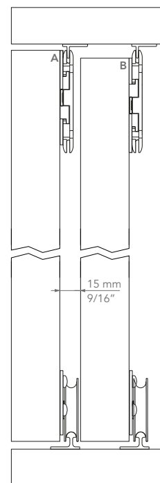
ROLL 52
