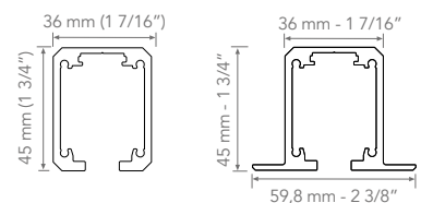
SLID 150
