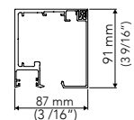
ROLLGLASS+ 150 TOP
