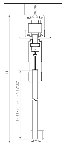
EMPOTRADO / RECESSED PERFIL TOP / TOP TRACK
