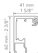
ROLLGLASS AUTO 40
