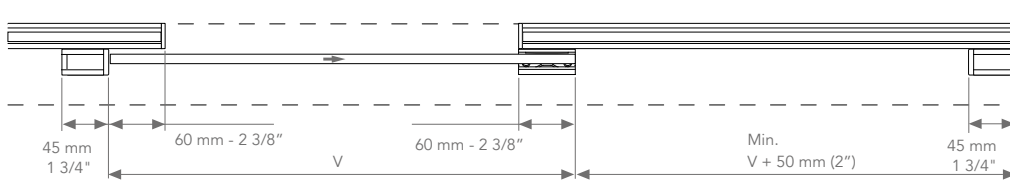
(VIDRIO FIJO / FIXED GLASS)
