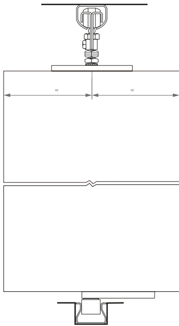
PL 40 C
