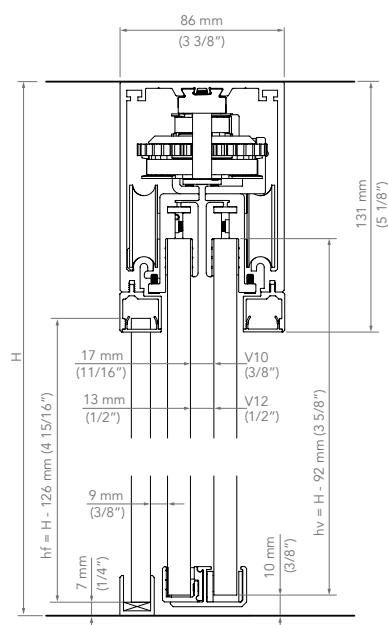
CON VIDRIO FIJO / WITH FIXED GLASS
