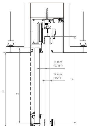
ROLLGLASS+ 150 TOP
