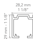
NK 60-85
