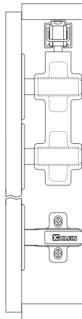
NK PAR 25
