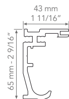
KT 200
