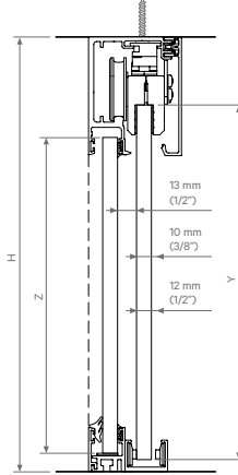
ROLLGLASS+ 150
