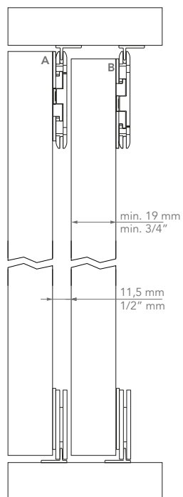
ROLL 45
