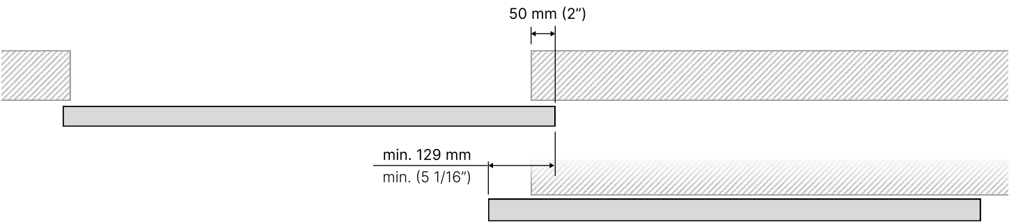
Puerta Centrada Door Centered
