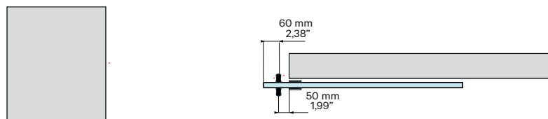
4 Puerta contra pared (Posición abierta) | Door against the wall (Opened position) | Porte contre mur ( Poste ouvert)
