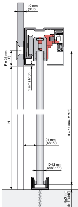
FIXED GLASS 3/8" / VIDRIO FIJO 10 mm
