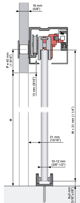
FIXED GLASS 5/8" / VIDRIO FIJO 16 mm
