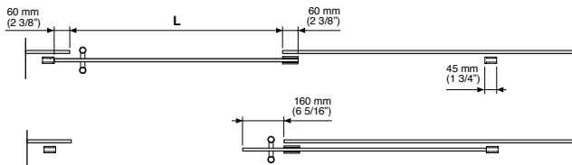
FIXED GLASS 3/8" / VIDRIO FIJO 10 mm
