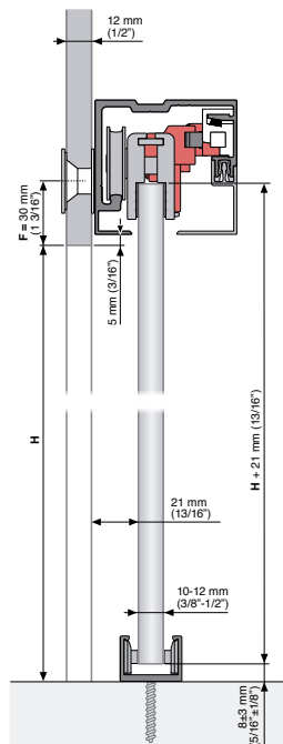
FIXED GLASS 1/2" / VIDRIO FIJO 12 mm
