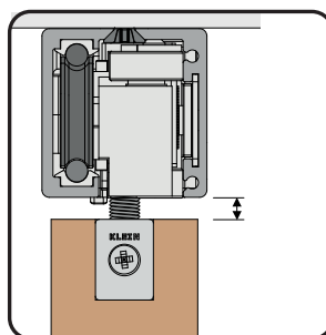
SANS VERROU 6 \pm 2 \text{ mm} ( 1/4'' \pm 1/16'' )
