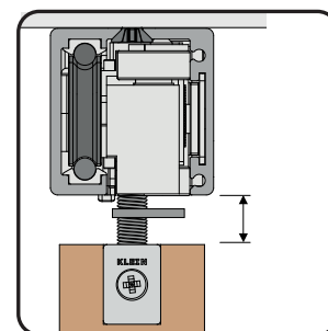
AVEC VERROU 11 \pm 2 \text{ mm} ( 7/16'' \pm 1/16'' )
