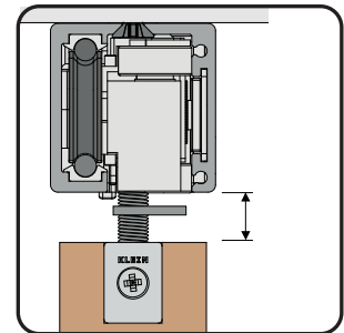
AVEC VERROU 11 \pm 2 \text{ mm } (7/16'' \pm 1/16'')
